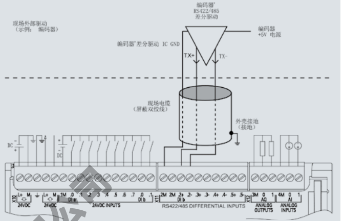
差分输入示意图
